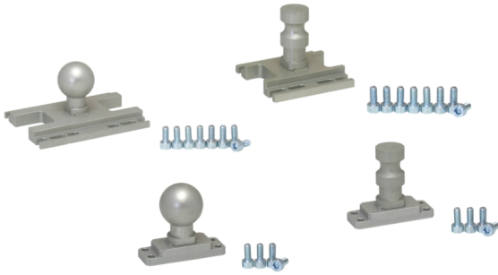
Sistema de soporte garras magnéticas SGM
